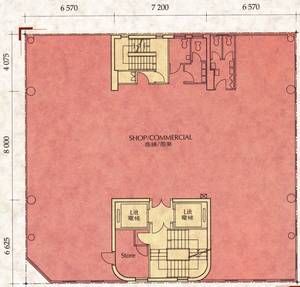
2ND FLOOR PLAN 二樓平面圖
